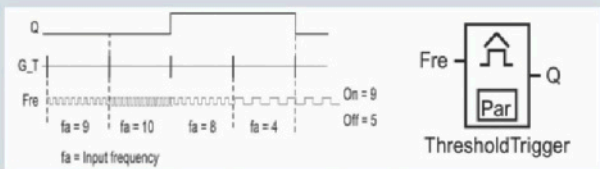
Schwellwertschalter
