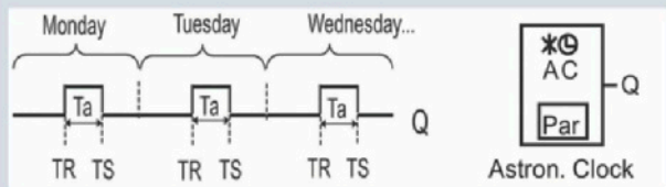
Astronomische Uhr
