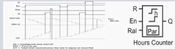
Betriebsstundenzähler
