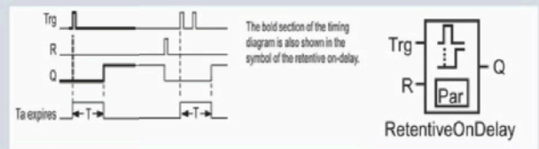
Speichernde Einschaltverzögerung
