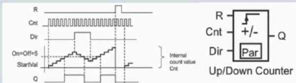
Vor-/Rückwärtszähler
