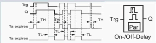
Ein-/Ausschaltverzögerung
