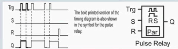
Stromstoßrelais
