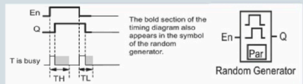
Zufallsgenerator
