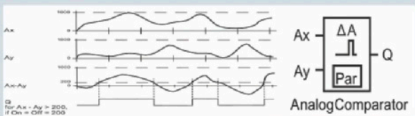
Analogkomparator
