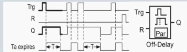
Ausschaltverzögerung
