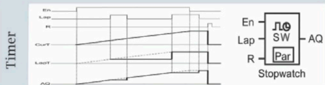
Stoppuhr
