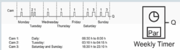
Wochenschaltuhr
