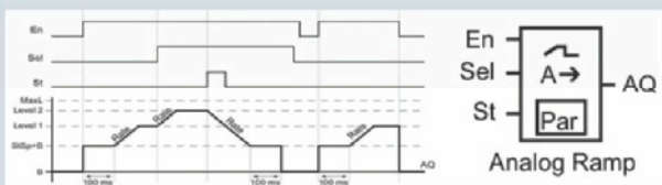
Analogrampe
