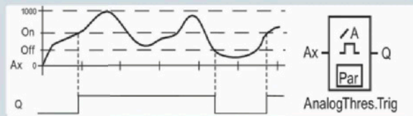
Analoger Schwellwertschalter
