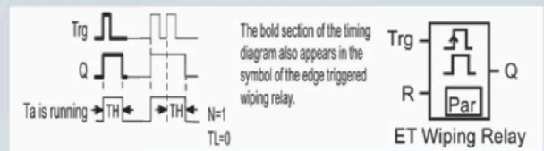
Wischrelais, flankengetriggert
