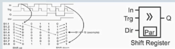
Schieberegister
