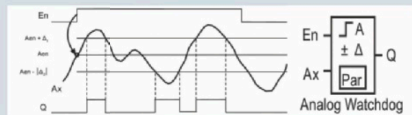
Analogwertüberwachung
