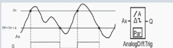
Analoger Differenz-Schwellwertschalter
