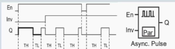
Impulsgeber
