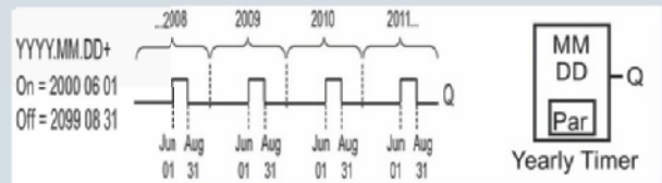
Jahresschaltuhr
