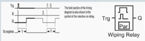
Wischrelais/Impulsausgabe
