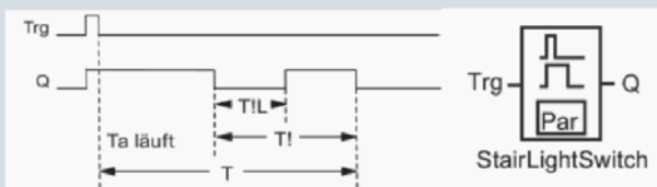
Treppenlichtschalter
