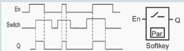
Softwareschalter
