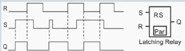
Selbhalterelais
